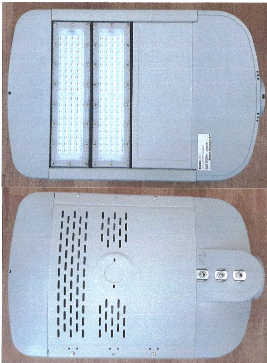
Рисунок 3 – Фотографии образца светильник светодиодный PсCOOLER BP-001-0018 (60Вт)
