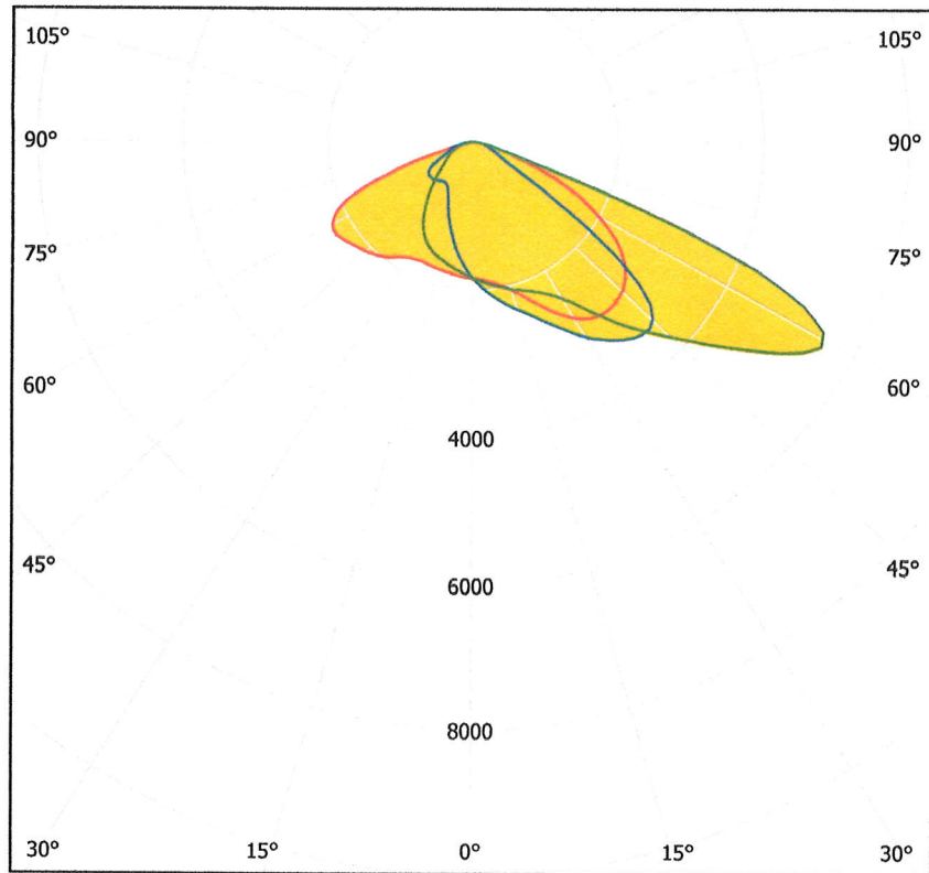
Рисунок 1 – КСС образца светильник светодиодный PsCOOLER BP-001-0018 (60Вт) в поперечной (C0-C180) (красная кривая), продольной (C90-C270) (синяя кривая) плоскостях и плоскости максимальной силы света (C150-C330) (зеленая кривая)
